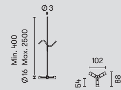
71-8251-05-05 Y-Steckverbinder | Connettore Y | У-образный соединитель
