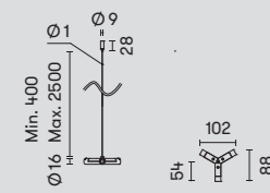
71-8257-05-05 Y-Steckverbinder | Connettore Y | У-образный соединитель
