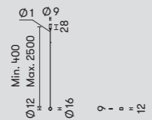
71-8264-05-05 Zubehör zur Verbindung von Strukturen Accessori di unione tra strutture Аксессуар для соединения структур
