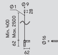
71-8260-05-05 Vertikaler 90°-Steckverbinder | Connettore 90° verticale | Соединитель 90°, вертикальный
