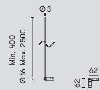
71-8254-05-05 Horizontaler 90°-Steckverbinder | Connettore 90° orizzontale | Соединитель 90°, горизонтальный
