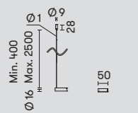
71-8263-05-05 Linearer End-Steckverbinder | Connecteur linéaire fina | Линейный соединитель концевой
