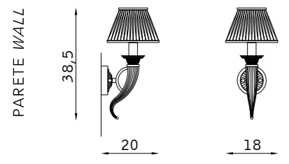
32519 1 x E14 30W
