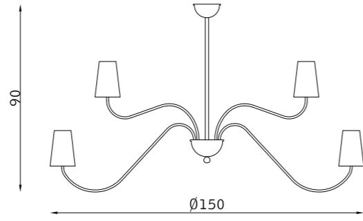
31193 18 x E14 9W
