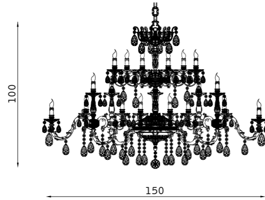
32539 28 x E14 30W
