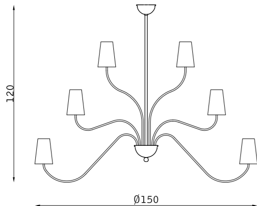
31194 21 x E14 9W
