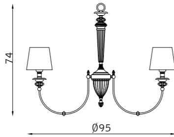
10363/S8 8 x E27 30W
