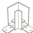
ST015.422.14 ■ ЧЕРНЫЙ ST015.522.14 □ БЕЛЫЙ УГОЛ-СОЕДИНИТЕЛЬ L78 × W78 × H57 MM
