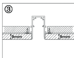
Схема монтажа
