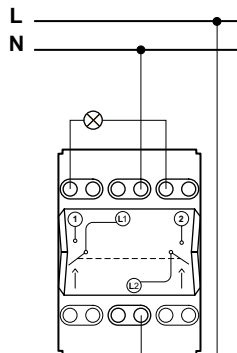
Двухполюсный переключатель
