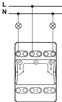
Двухклавишный выключатель
