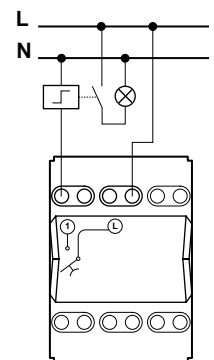
Кнопочный выключатель
