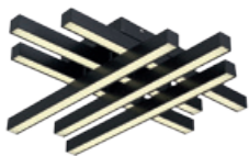
SL933.402.06 черный | черный | белый ■ ■ ■ LED 1 × 36 W 3000 K / 4000 K / 6000 K 2736 lm ↗ 600 | ↓ 125 | ↔ 600 металл | металл | акрил
