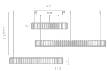
4 1135/17 SP-106
