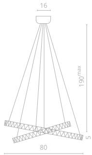
1 1030/17 SP-144 Ø80 | 195 | 190 max LED 1x52W 3800Lm 3000K CRI≥80 Bulb incl.
