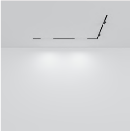
Профиль-трек SMART ONE TR2023-BK - 1 шт Угловой элемент 90° Denkirs TR2026-BK - 1 шт Комплект соединителей прямых TR3043-AL - 2 шт Комплект торцевых заглушек Denkirs TR2025-BK - 1 шт Уголок регулируемый для закладных профилей Denkirs TR3045-AL - 5 шт Гибкий коннектор Denkirs TR2103-BK - 1 шт Подвод питания Denkirs TR2100-BK - 1 шт Пульт управления Denkirs DK7300-BK - 1 шт Трековый светильник Denkirs DK8004-BK - 2 шт Трековый светильник Denkirs DK8010-BK - 2 шт
