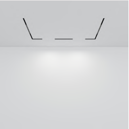
Профиль-трек SMART ONE TR2022-BK - 2шт Угловой элемент 90° Denkirs TR2026-BK - 2шт Комплект соединителей прямых TR3043-AL - 4шт Комплект торцевых заглушек Denkirs TR2025-BK - 1шт Уголок регулируемый для закладных профилей Denkirs TR3045-AL - 7шт Гибкий коннектор Denkirs TR2103-BK - 2шт Подвод питания Denkirs TR2100-BK - 1шт Пульт управления Denkirs DK7300-BK - 1шт Трековый светильник Denkirs DK8004-BK - 2шт Трековый светильник Denkirs DK8002-BK - 2шт
