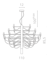
1 8030/02 LM-50 ∅110 | 86 | 100 max 50x15W E14 Bulb incl.
