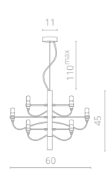
3 8030/02 LM-18 ∅60 | 45 | 110 max 18x15W E14 Bulb incl.
