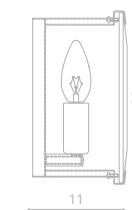
3 1100/02 AP-1 ↔11 | ↗11 | ↓20 ⚡ 1x60W E14
