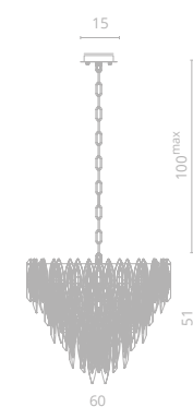
1 3509/01 LM-12 ∅60 | 146 | 100 max ⚡ 12x60W E14 ⚙️ 20
