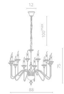
2 1021/02 LM-12 ∅88 | 175 | 100 max 12x60W E14
