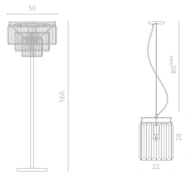
9 3001/02 PN-6 10 3001/02 SP-1 ø50 | 160 ø22 | 28 | 100 max 6x40W E14 1x75W E27 25
