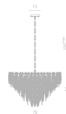
2 3509/01 LM-15 ∅78 | 151 | 100 max ⚡ 15x60W E14 ⚙️ 35
