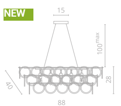
6 7566/01 SP-13 ↔88 | ↗40 | ↓28 | 100 max ⚡ 13x40W E14
