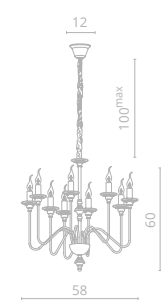
1 1021/02 LM-9 ∅58 | 160 | 100 max 9x60W E14
