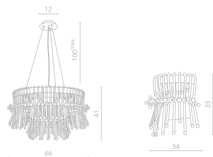
3 7565/01 SP-7 4 7565/01 AP-1 Ø66 | 41 | 100 max ↔34 | 20 | 33 ⚡ 7x60W E14 ⚡ 1x60W E14
