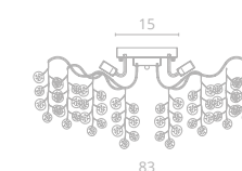
7 7288/26 PL-8 Ø83 | 137 8x40W E14
