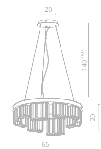
2 6817/02 SP-10 ∅65 | 120 | 140 max 10x40W G9
