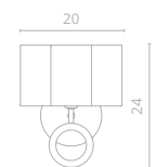
2 4069/02 AP-1 ↔20 | ↑17 | ↑24 ⚡ 1x40W E14
