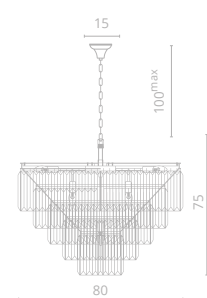
1 3005/23 SP-18 Ø80 | 75 | 100 max 18x60W E14 23
