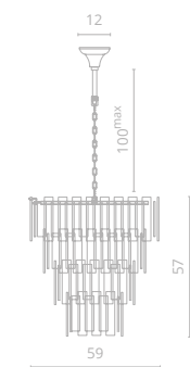
2 6005/17 LM-9 Ø59 | 57 | 100 max 9x40W E14 22
