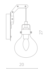
3 1001/16 AP-1 ↔12 | ↗20 | ↑27 ⚡ 1x40W E14
