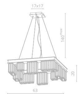
3 6817/02 SP-12 ↔63 | ↗63 | 120 | 140 max 12x40W G9
