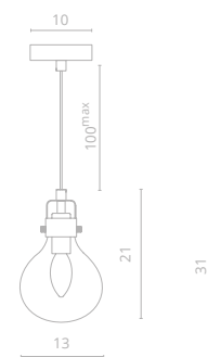
2 1001/16 SP-1 ∅13 | ↑21 | 100 max ⚡ 1x40W E14
