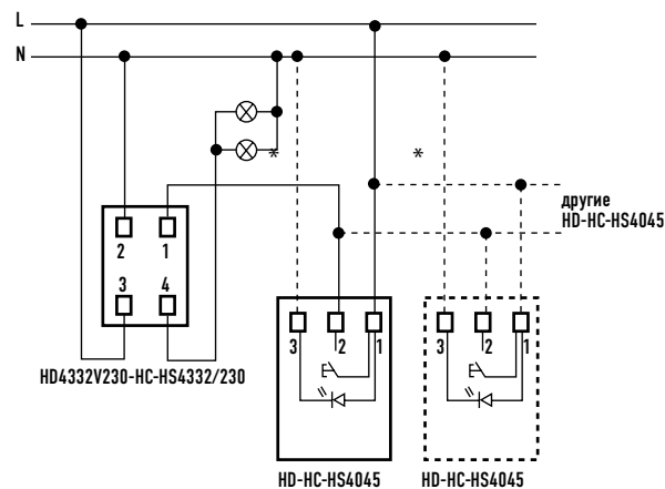
4-проводное подключение
