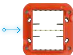
H4726 (на винтах) межосевое расстояние крепежных винтов 46×83,5 мм
