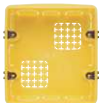
506E (108×118×51,5 мм) для бетонных стен
