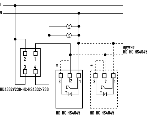
3-проводное подключение
