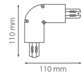
соединитель трехфазный накладной L-образный
