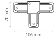
соединитель однофазный накладной T-образный
