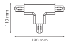
соединитель трехфазный накладной T-образный
