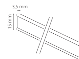
Трек DUE 48V 5 метров
