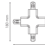
соединитель трехфазный накладной X-образный
