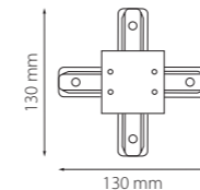
соединитель однофазный встраиваемый X-образный
