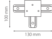
соединитель однофазный встраиваемый T-образный
